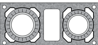
двухходовой с вентиляционным каналом
