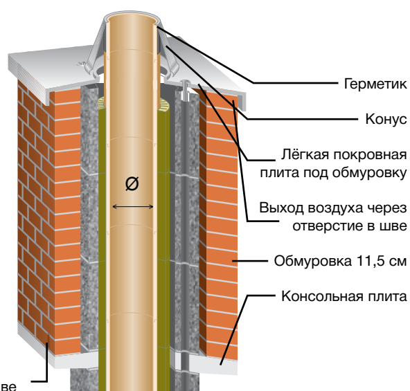
Выполняемая по месту обмуровка на консольной плите
