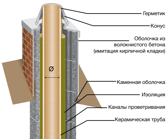
Оболочка дымовой трубы из волокнистого бетона с имитацией кирпичной кладки
